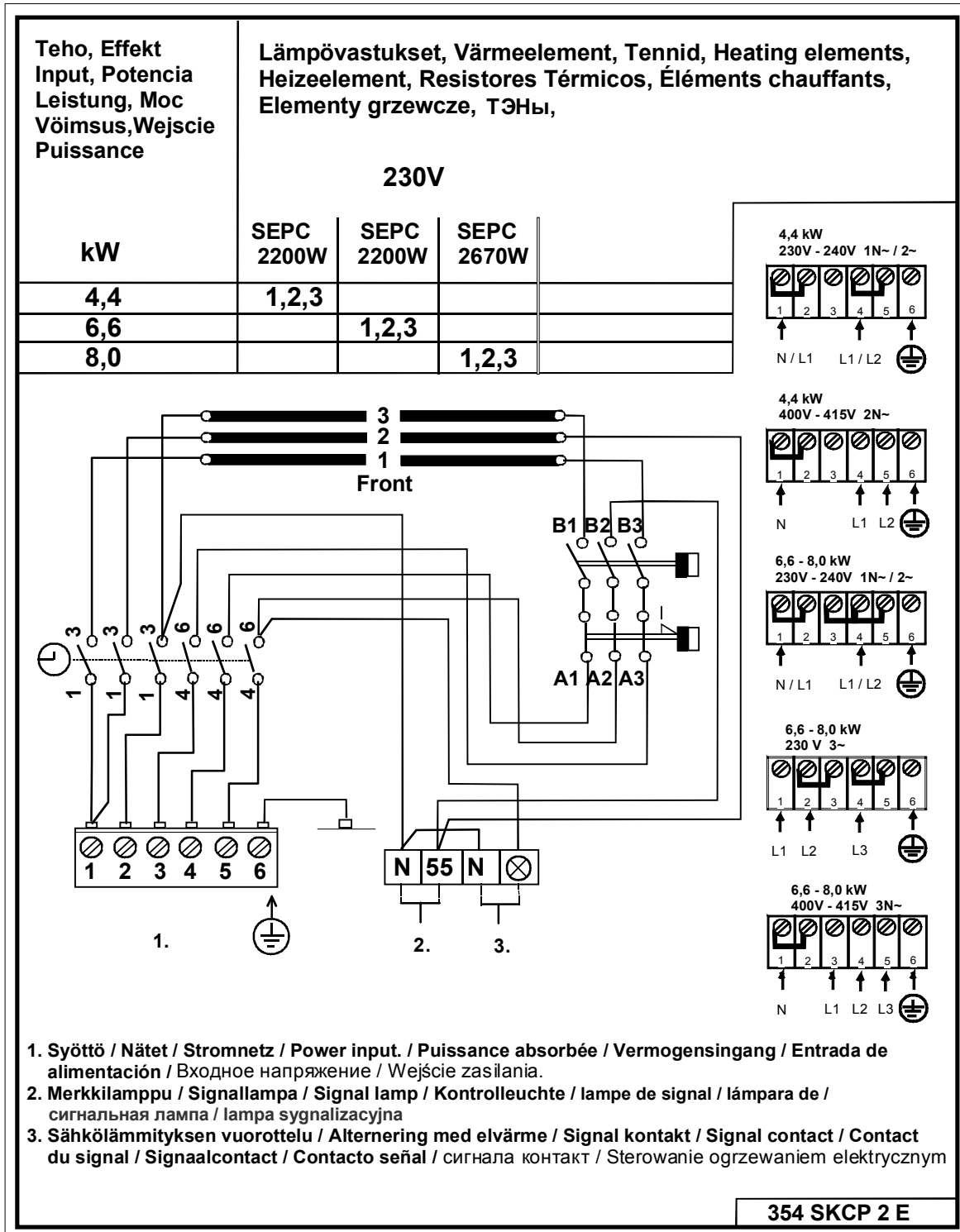
Bild 4 Kopplingschema
