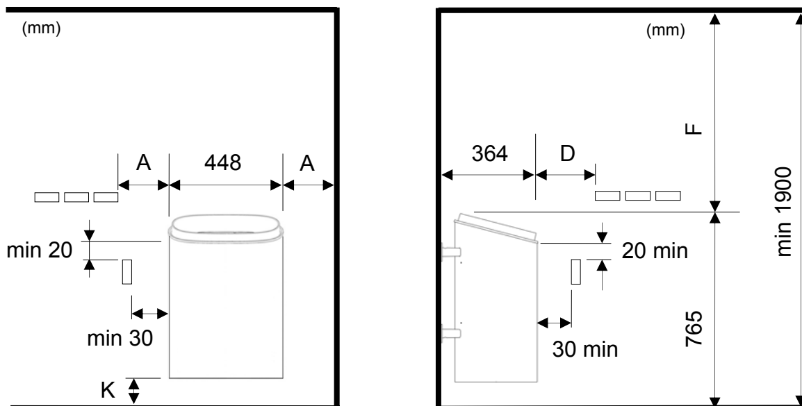
Bild 2 Skyddsavstånd
